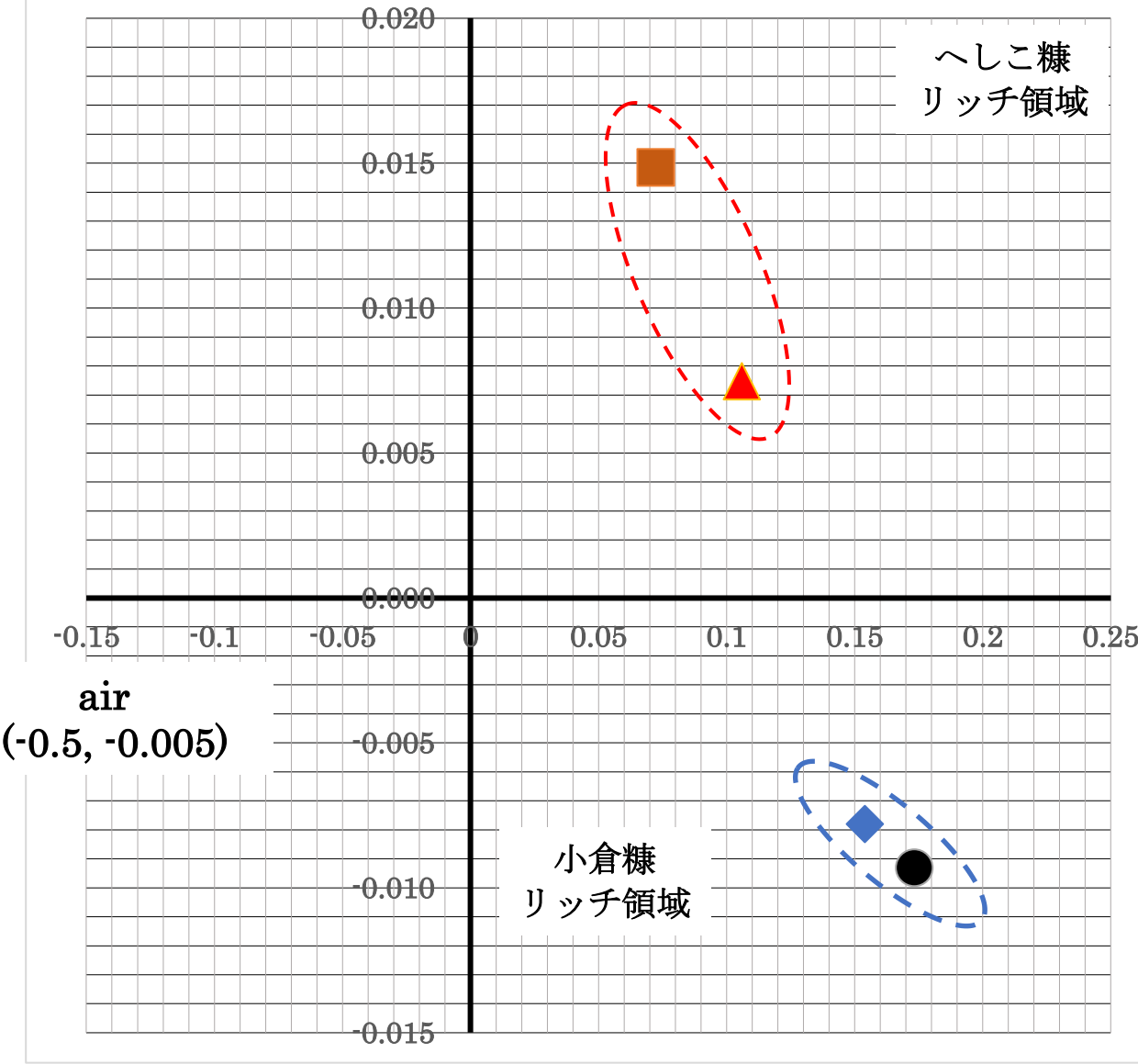
2022年の第5回交流会の糠炊き官能評価結果の主成分分析結果（電子嗅覚装置併用：水産大）
